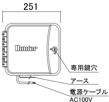
正面
