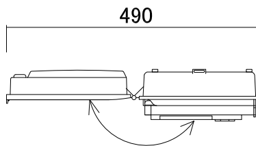
上面(操作時)
