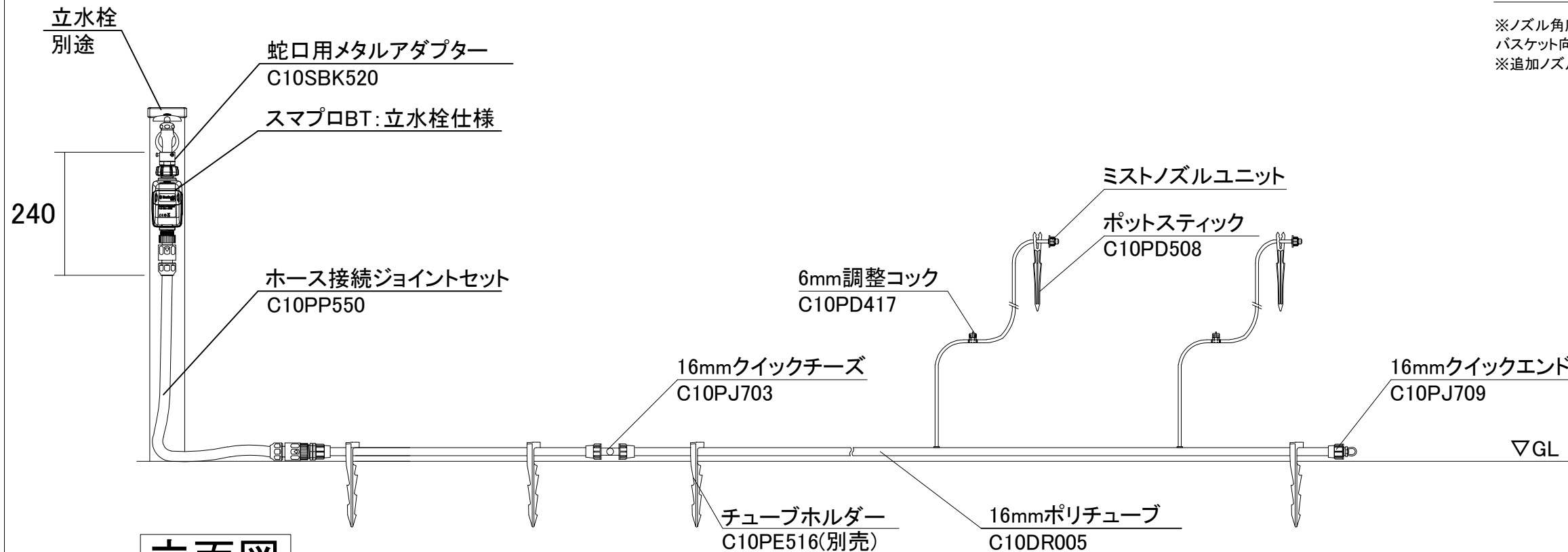
立面図
