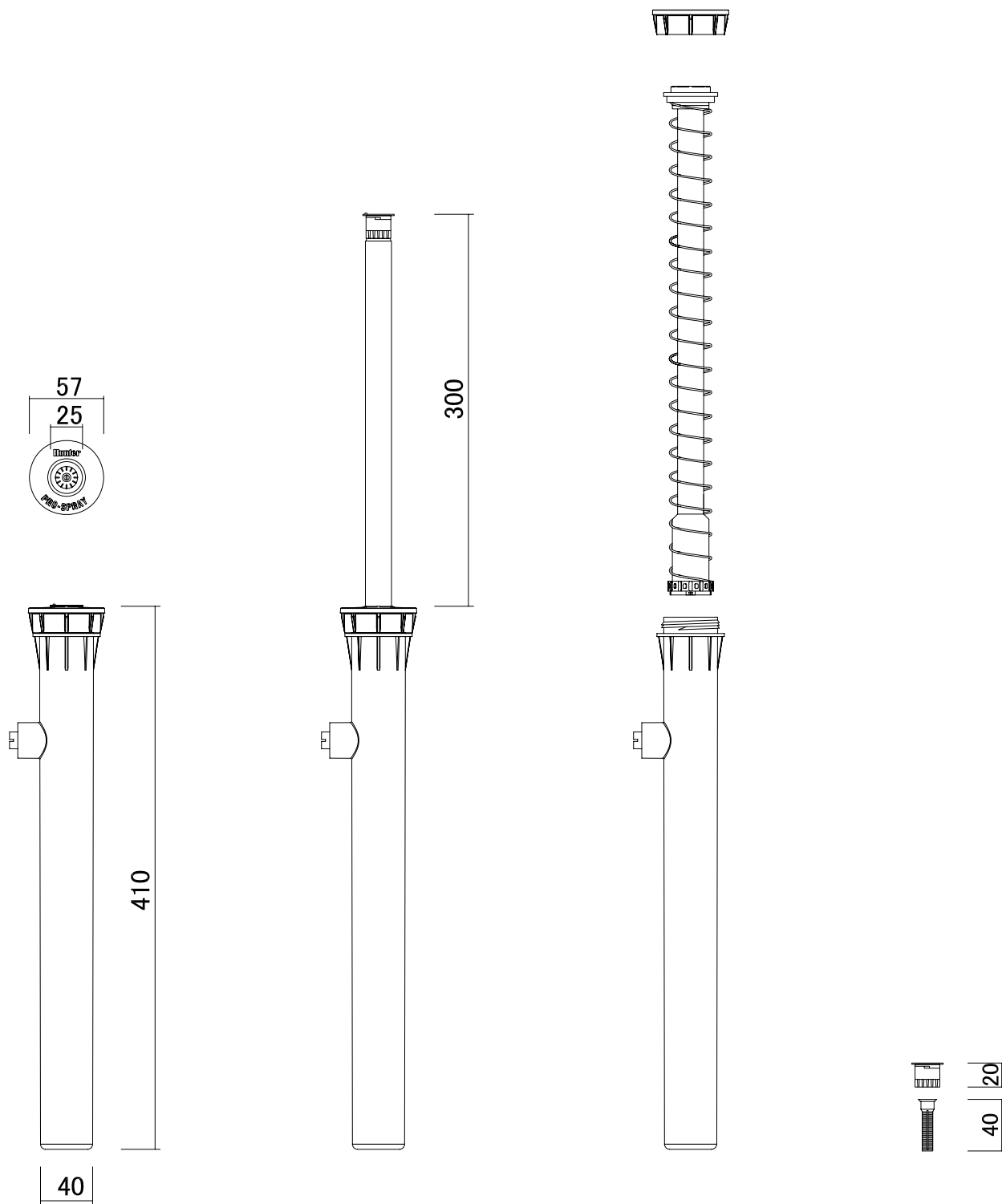
立面図
