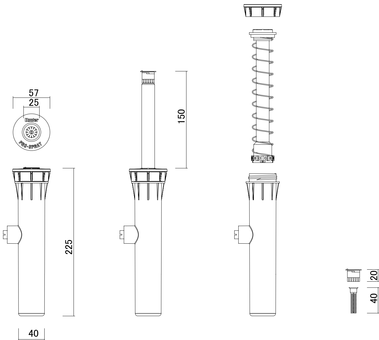
立面図
