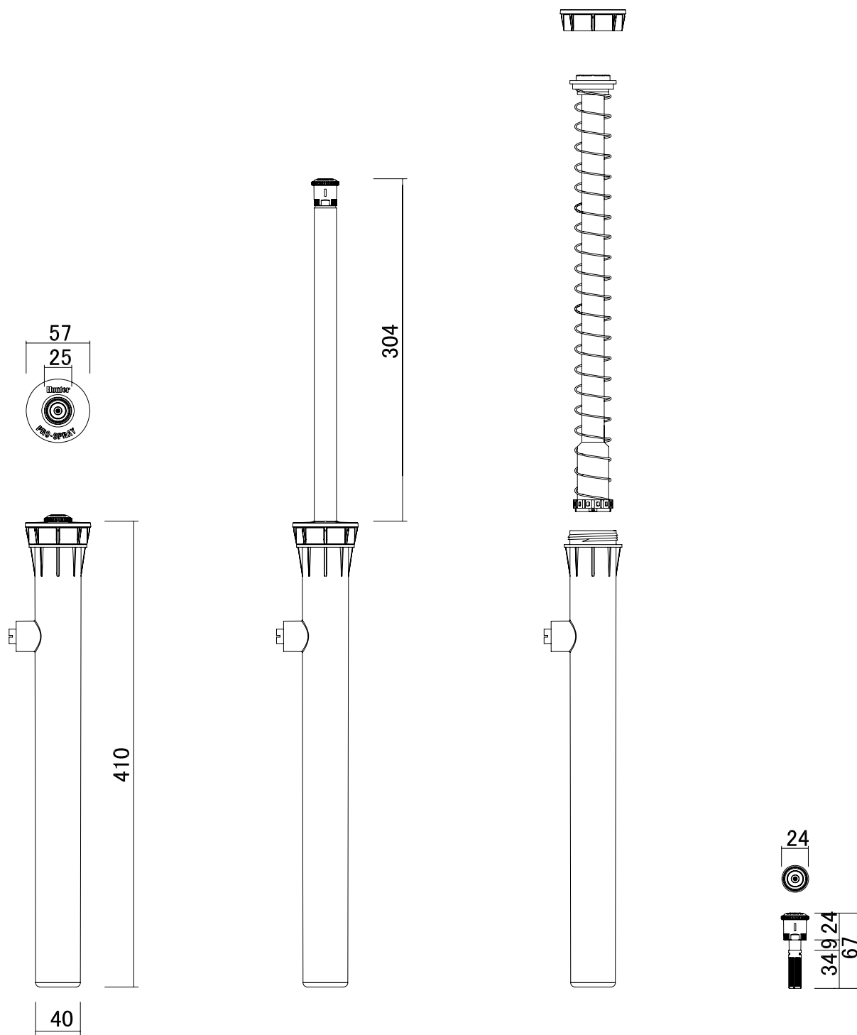
立面図
