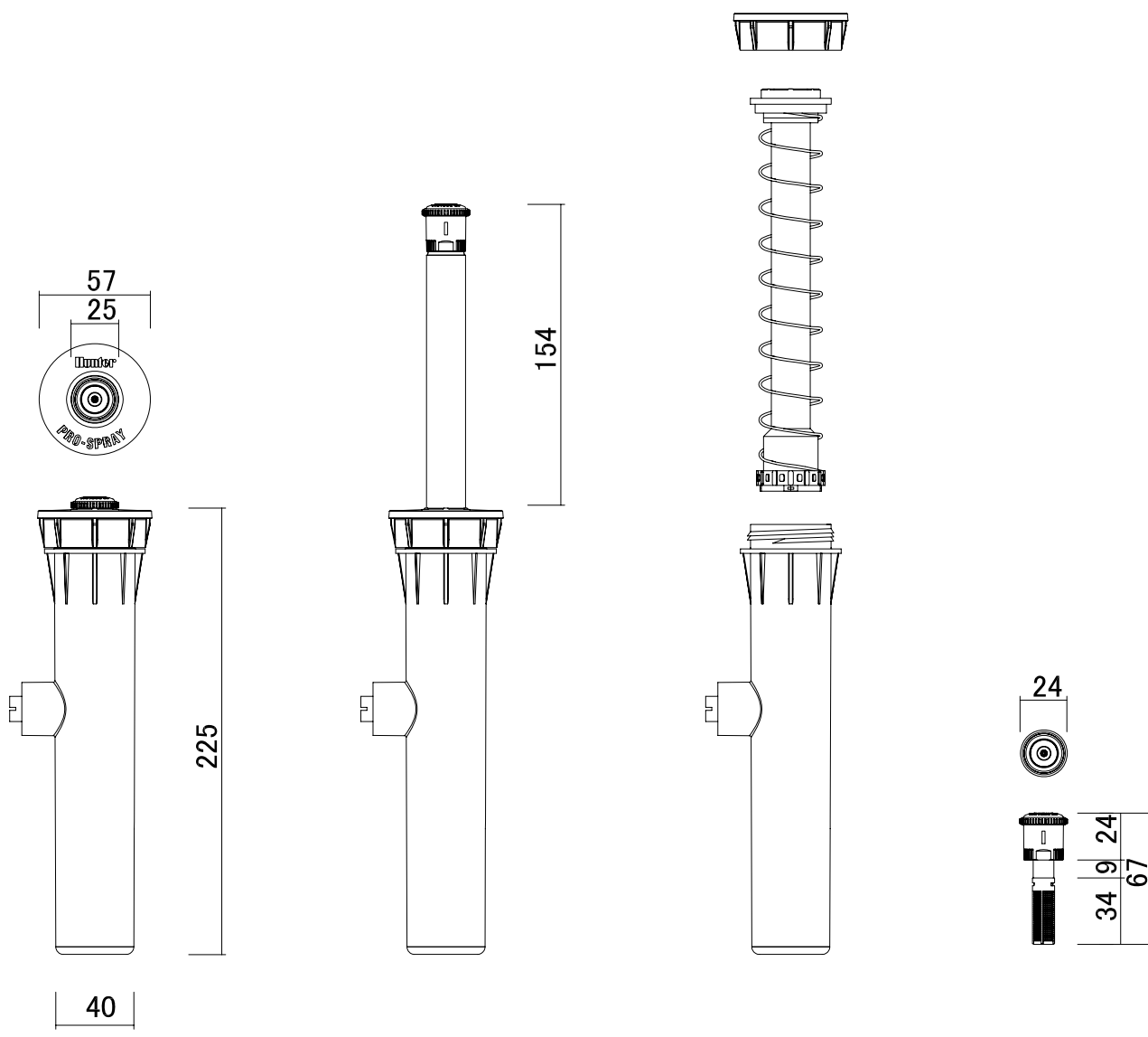
立面図 ポップアップ時 分解図 付属ノズル
